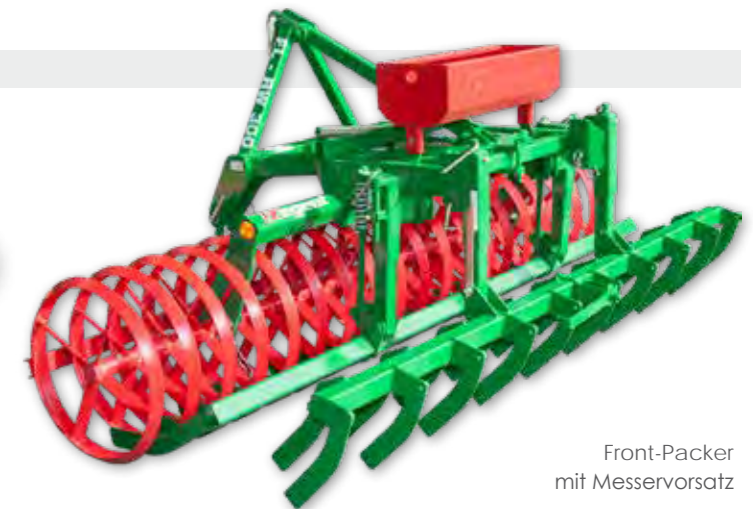
Front-Packer mit zweireihigem Federzahnvorsatz
